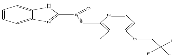
Dexlansoprazole
